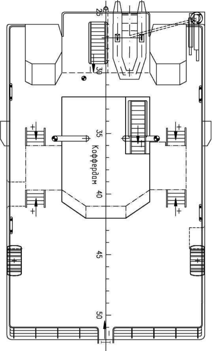
Палуба рубки
