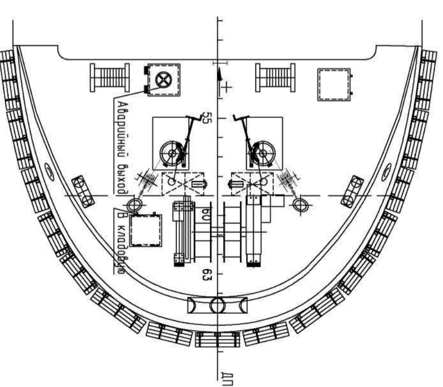
Палуба вака
